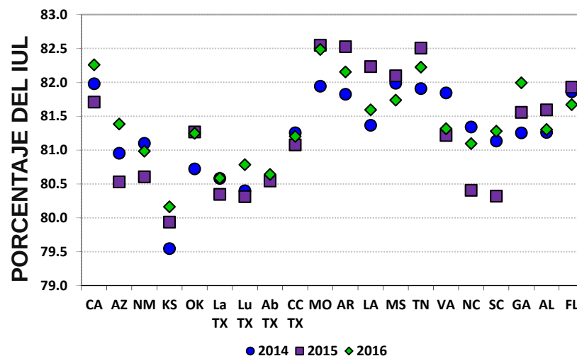
UNIFORMIDAD DE LONGITUD PROMEDIO
