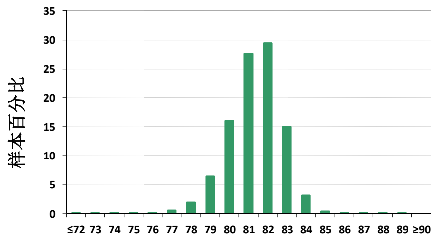
美国陆地棉长度整齐度分布图
